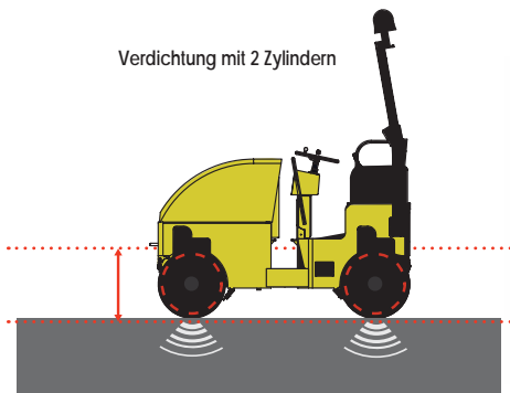
Vibrierende Zylinder
